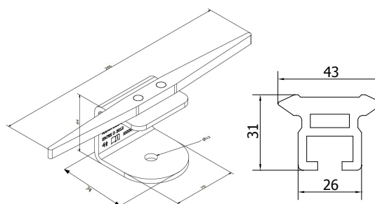
Soporte de raíl
